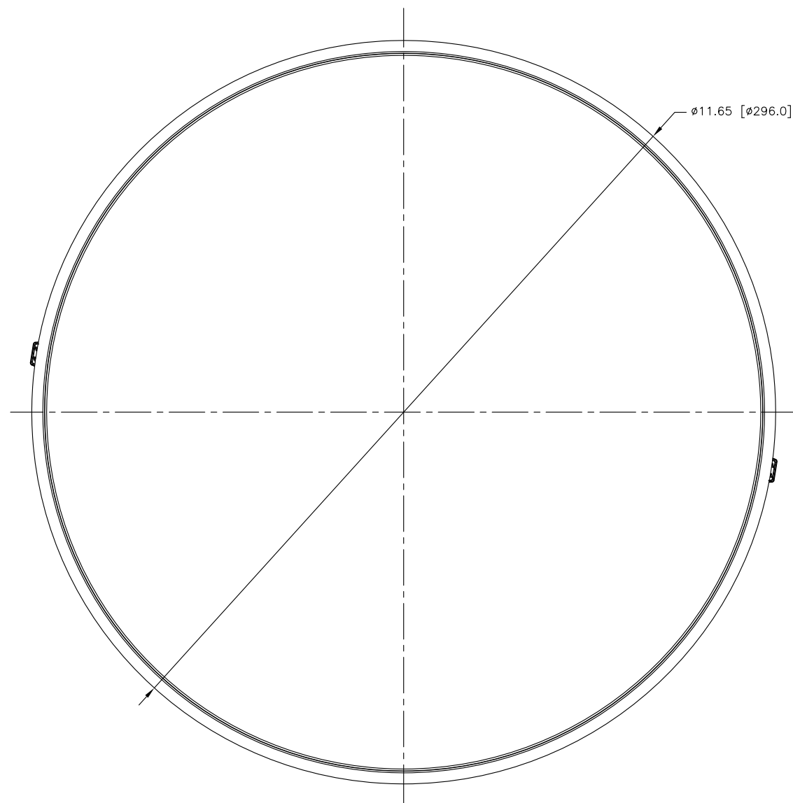
GRILLE
